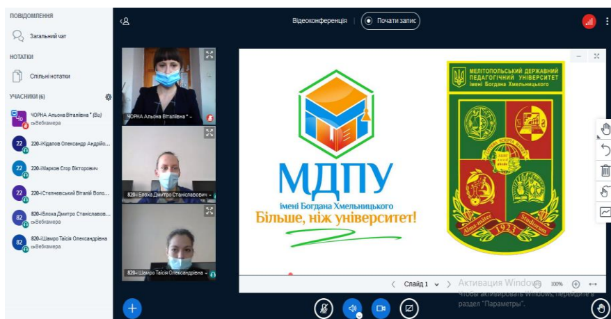
Рис.1.16. Відеоконференція BigBlueButton.
